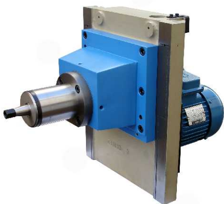
Cabeçote do rebolo
